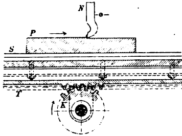
Č. 1731. Hoblovací stroj na kovy (pohybovací mechanismus pro předmět).
